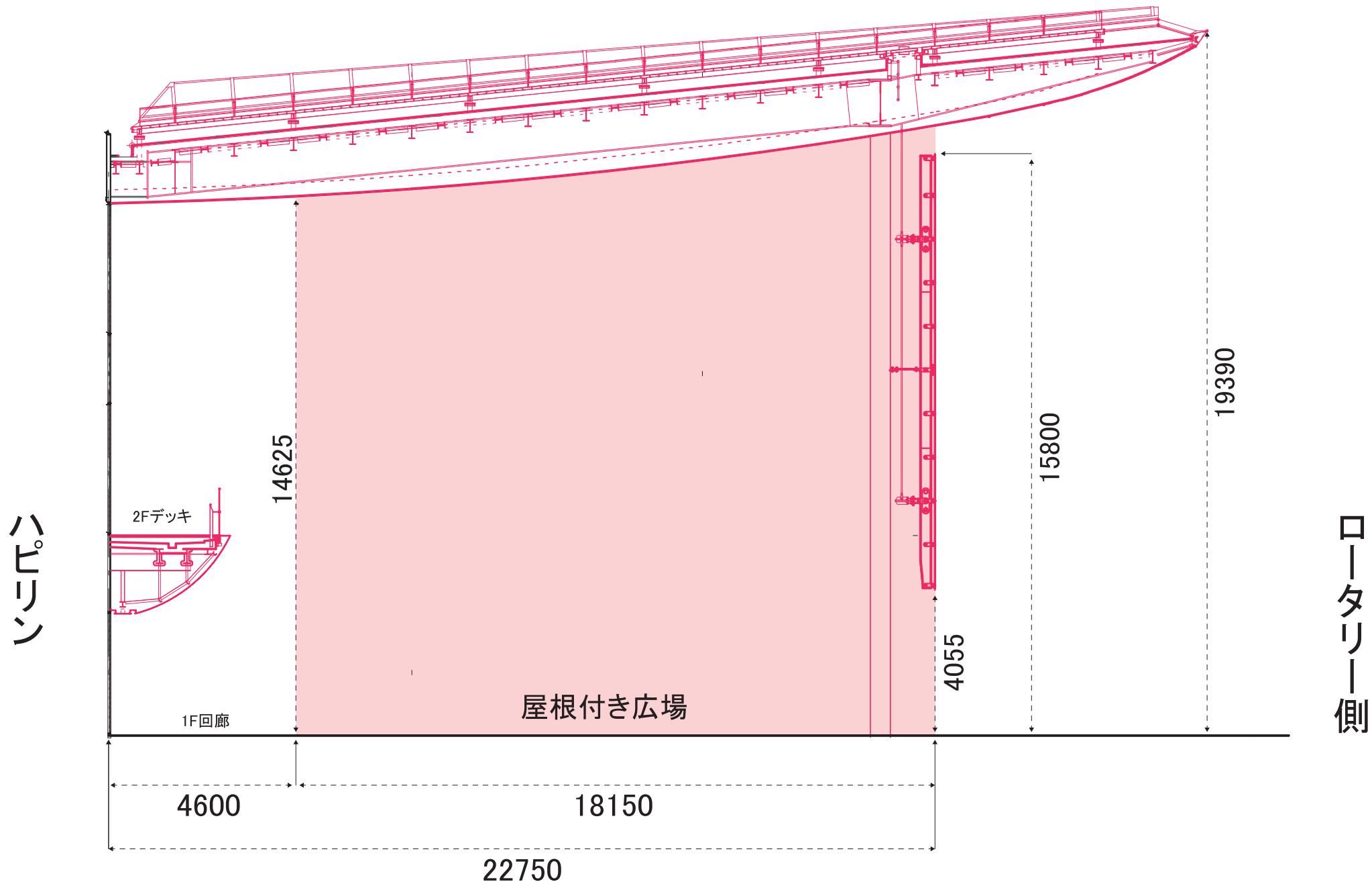
ハピテラス簡易断面図(単位:mm)
